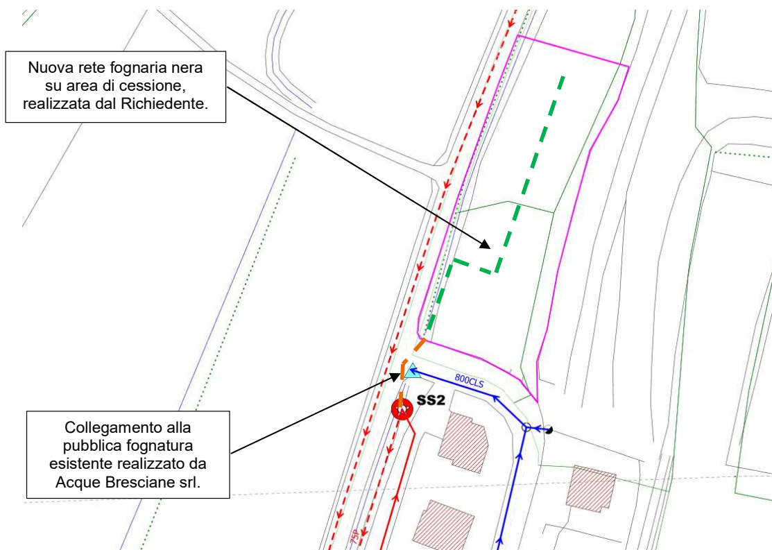
PL.01- Planimetria rete fognaria comunale.
