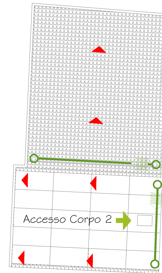
PIANTA FABBRICATO OGGETTO DI OPERE DI STRAORDINARIA MANUTENZIONE - Progetto 1: 100
