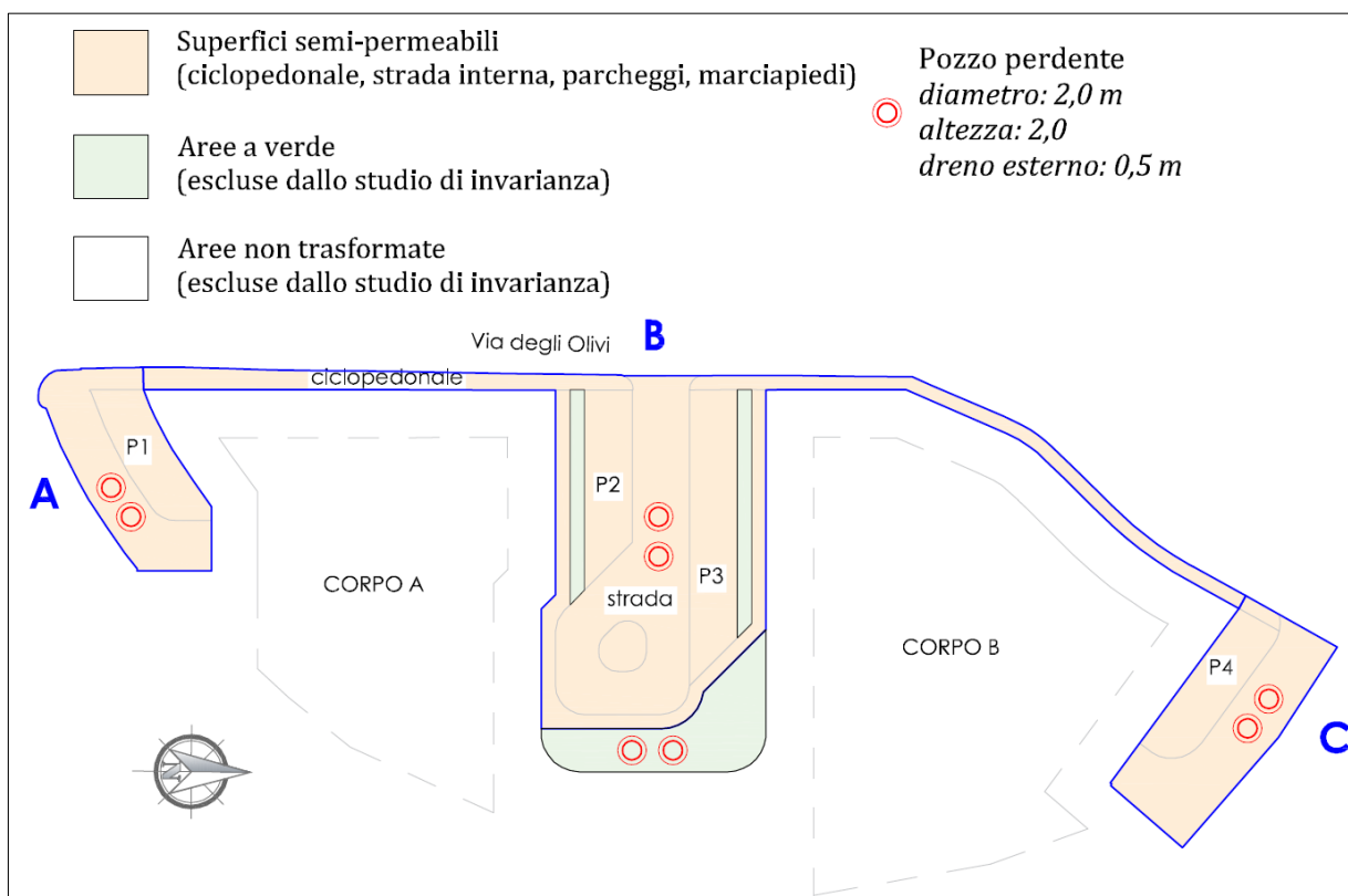
Fig. 6 - Planimetria di progetto con individuazione dei settori progettuali (A, B e C), delle nuove superfici semi-permeabili (arancio), le aree a verde (verde) e quelle non trasformate (bianco), e dell'ingombro delle opere di immagazzinamento e smaltimento delle acque progettuali.
