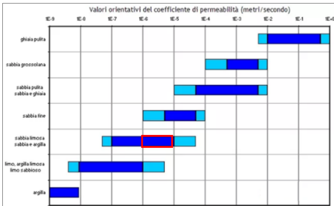
Fig. 9 - Valori indicativi del coefficiente di permeabilità.
