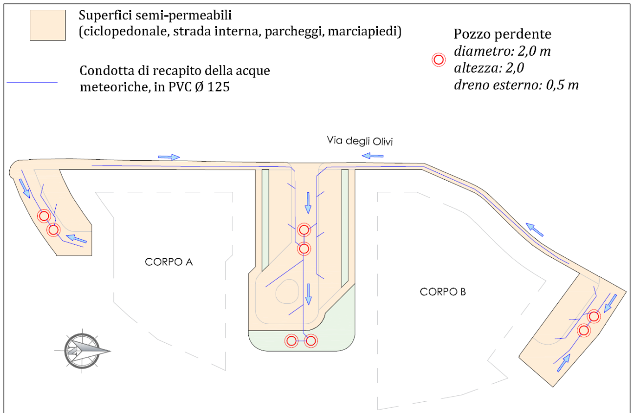
Fig. 11 - Individuazione del sistema di dispersione, costituito da n°9 pozzi perdenti, conformemente allo studio di invarianza idraulica.
