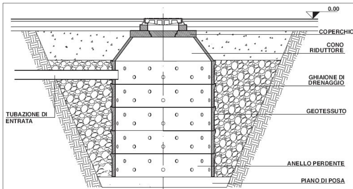
Fig. 10 - Schema costruttivo del pozzo perdente per lo smaltimento delle acque di prima pioggia, da realizzare fino a -2,0 m dal p.c.
